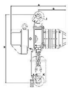
0.5 Ton - 10 Ton Electric Hoist
